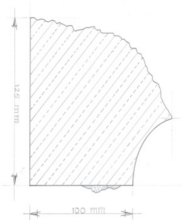
Doorsnede van vensterstijl uitgevoerd in mergelsteen
