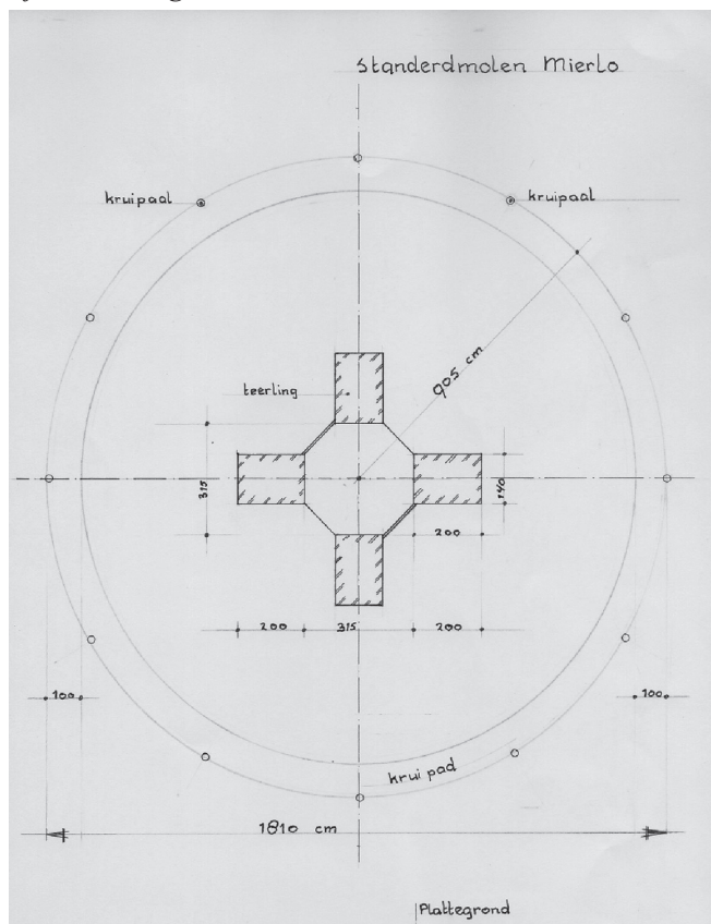
Afb. 4 Plattegrond
