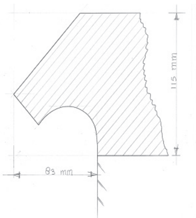
Gedeelte van regenlijst
