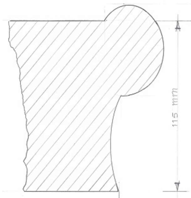
Muurafdek dik 60 mm.
